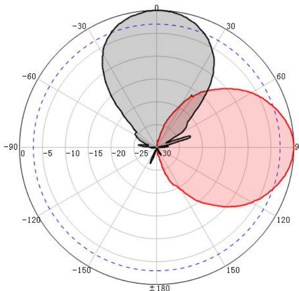
H-Pol- 6.6GHz
