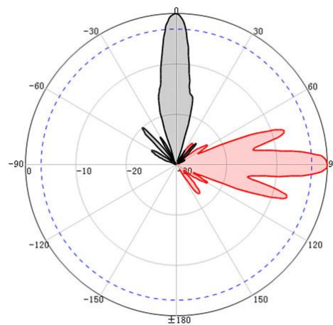
V-Pol
