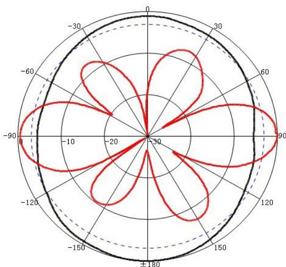
H-Pol @ 2450MHz
