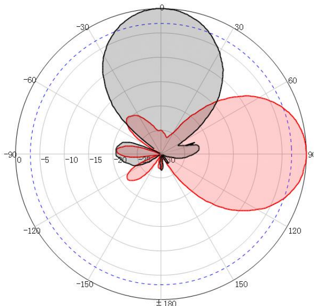
868MHz
