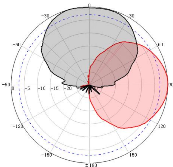
H-Pol- 6.6GHz
