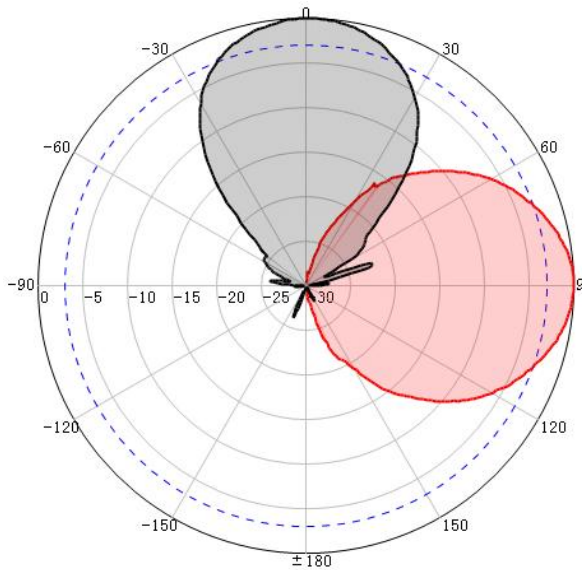
H-Pol- 6.6GHz
