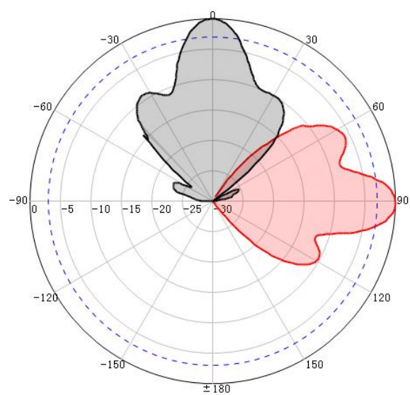
V-Pol– 6.6GHz
