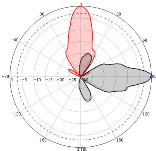
H-Pol.
