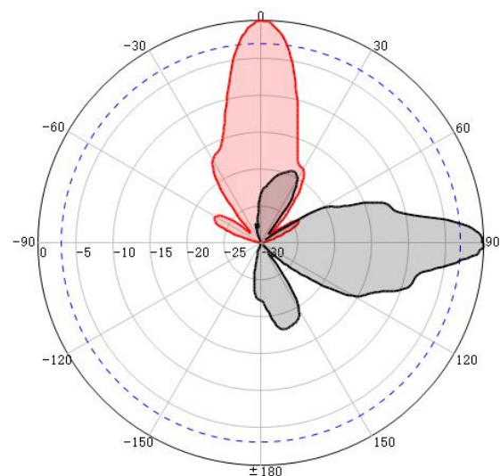
V-Pol.
