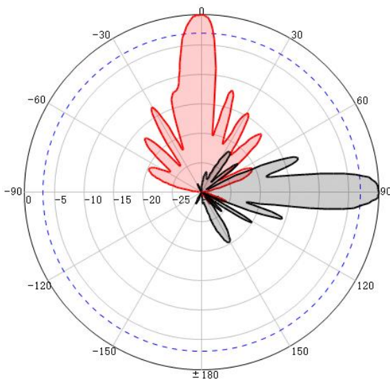
H-Pol
