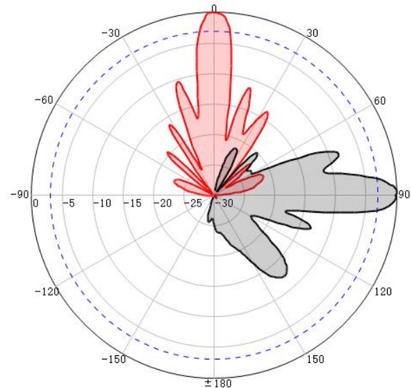
V-Pol
