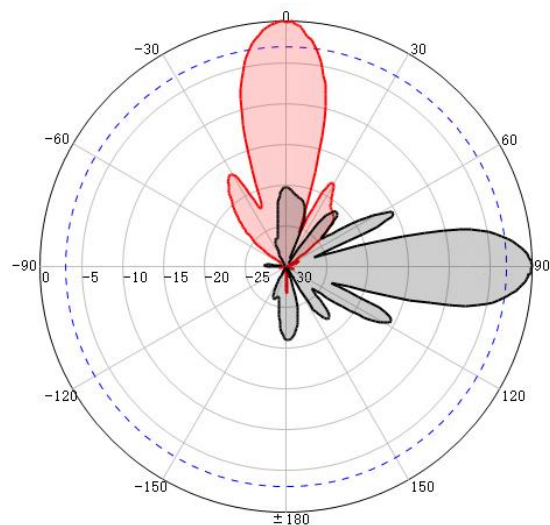
V-Pol@1710MHz
