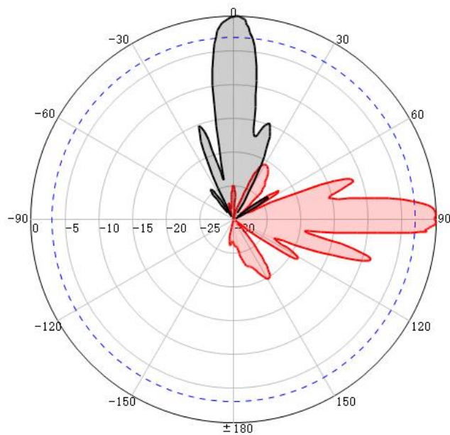
V-Pol@2700MHz
