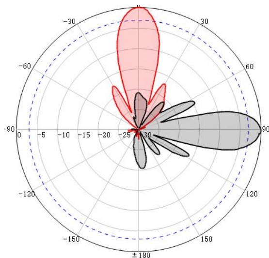
H-Pol@1710MHz
