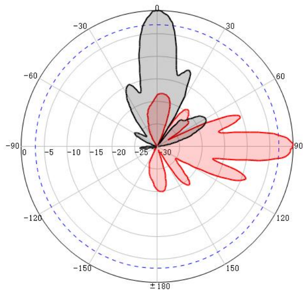
V-Pol@2200MHz
