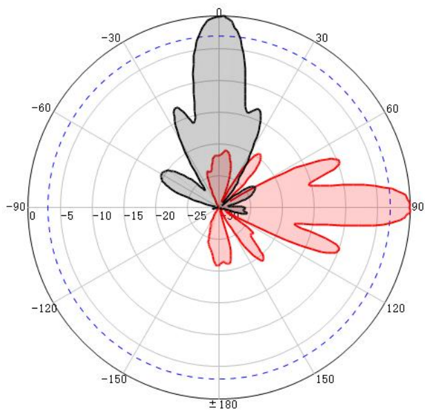
H-Pol@2200MHz
