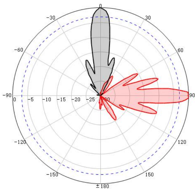
H-Pol@2700MHz
