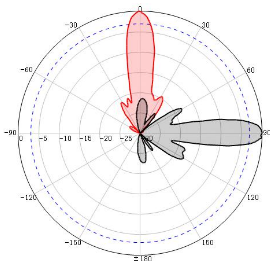
H-Pol@2700MHz
