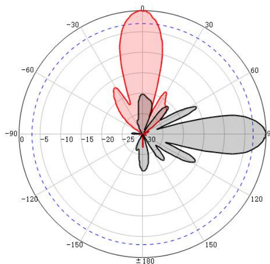
V-Pol@1710MHz
