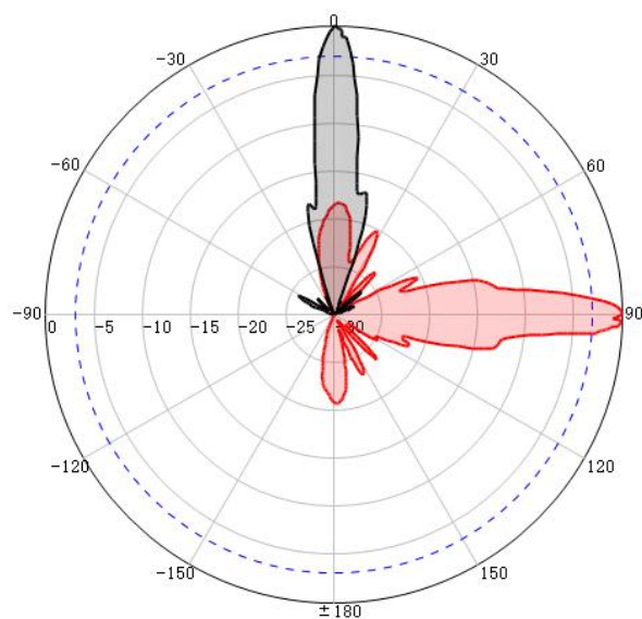
H-Pol@3500MHz
