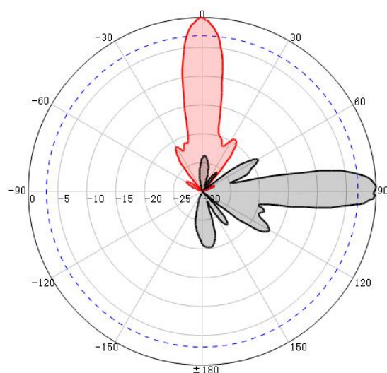
V-Pol@2700MHz
