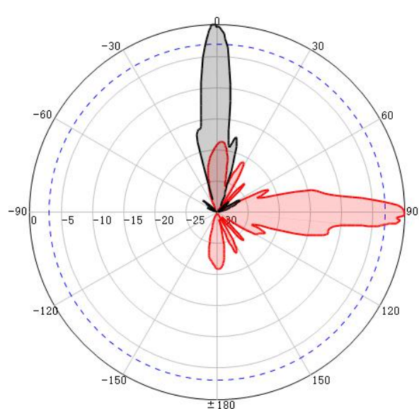
V-Pol@3500MHz
