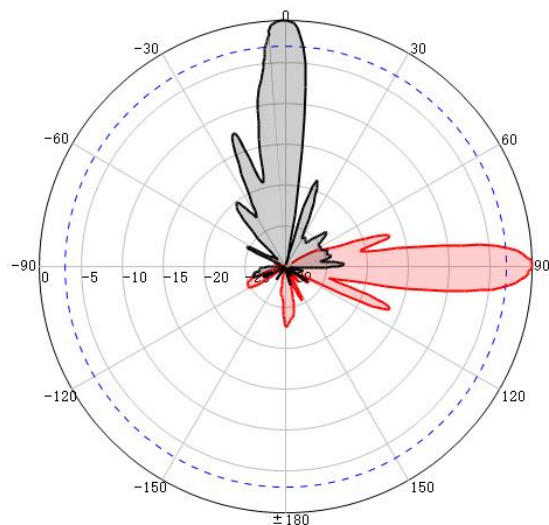
RHCP @4000MHz
