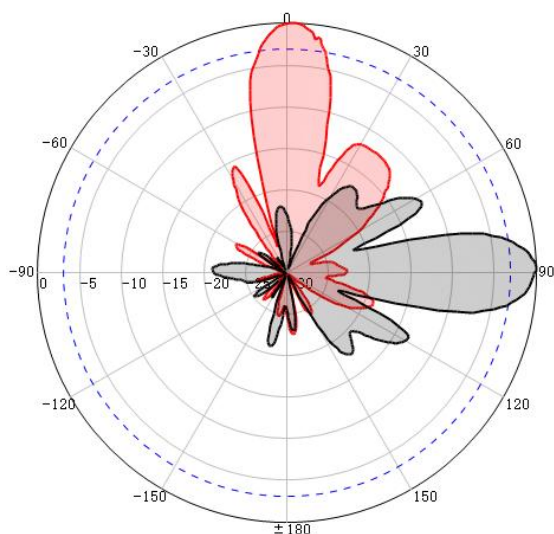
LHCP @1710MHz
