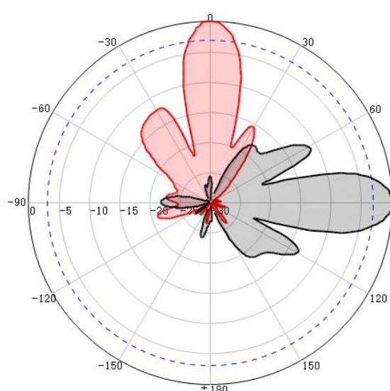
RHCP @1710MHz
