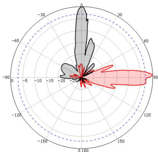
LHCP @4000MHz
