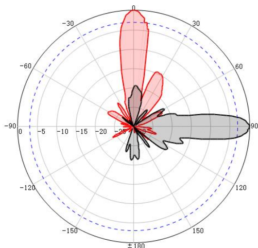
LHCP @2700MHz
