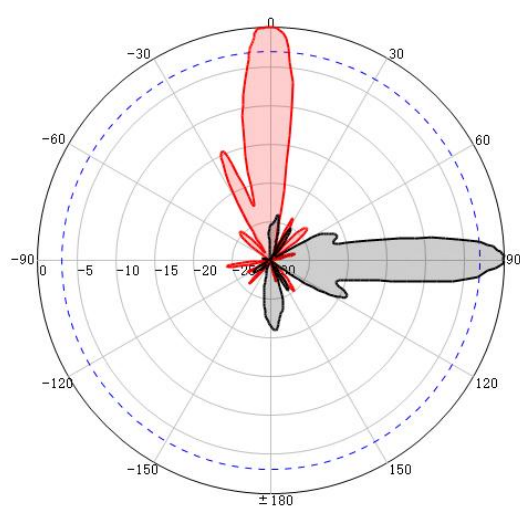
RHCP @3300MHz
