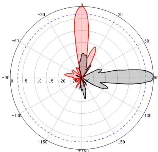
LHCP @3300MHz
