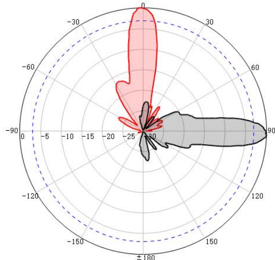
RHCP @2700MHz
