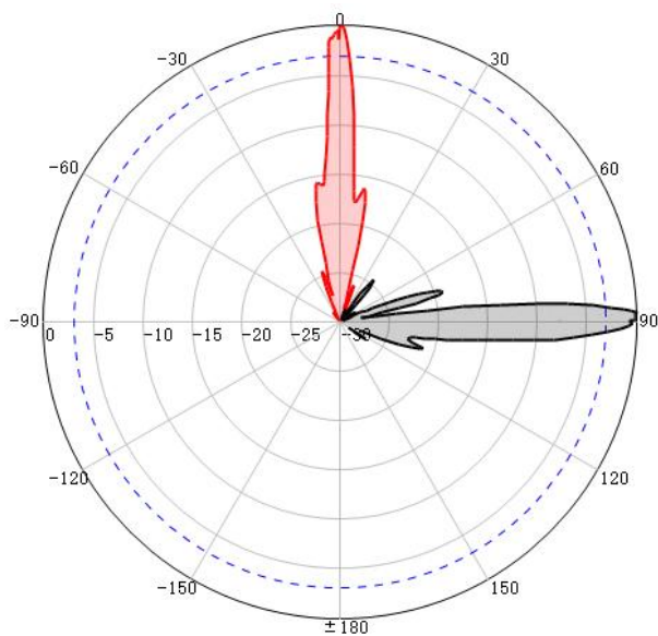
H-Pol@ 5.0 GHz
