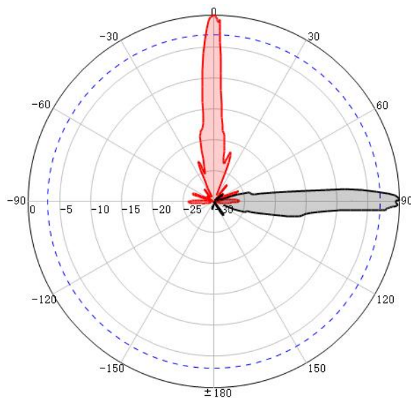
V-Pol@ 4.7GHz
