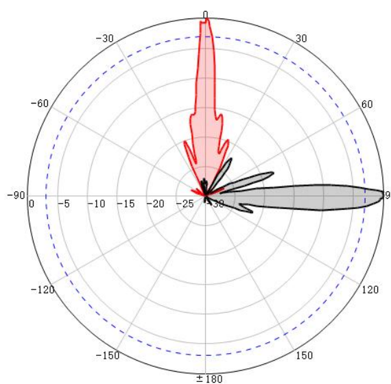
V-Pol@ 4.4GHz
