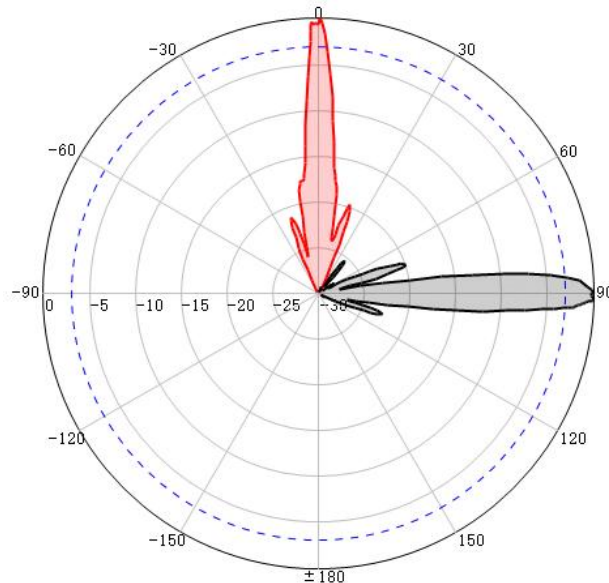
V-Pol@ 5.0 GHz
